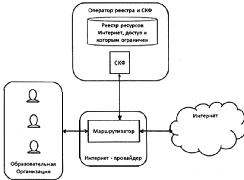
Рис.5. Схема работы контент-фильтрации при едином решении
