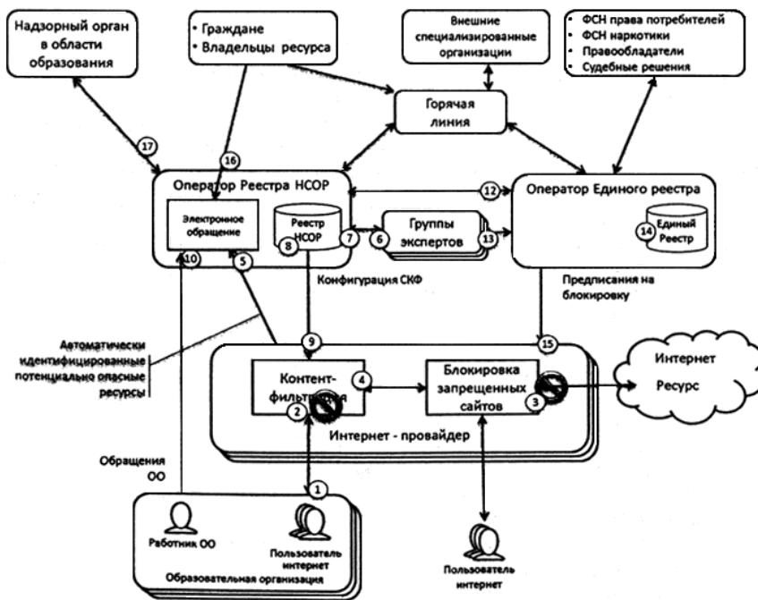
Рис.7. Схема процесса взаимодействия
